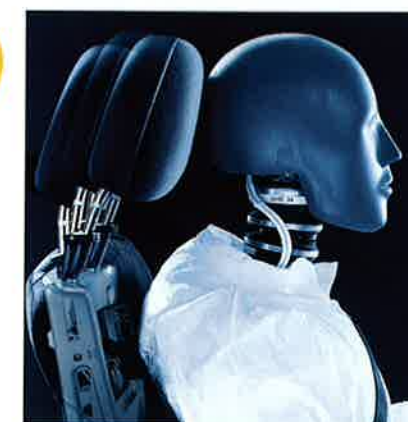
Aktive Kopfstützen
