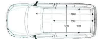
Alle Maße in mm (Kastenwagen)
